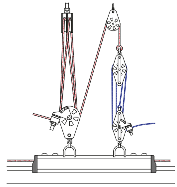
6:1 Mainsheet plus 24:1 fine tune
